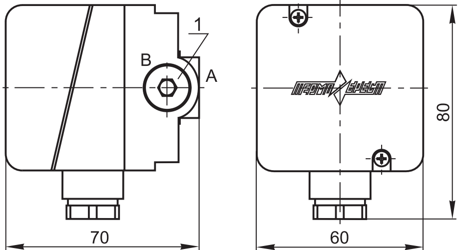
Рис. 25-1. Габаритные размеры датчиков-реле давления серии ДРД
