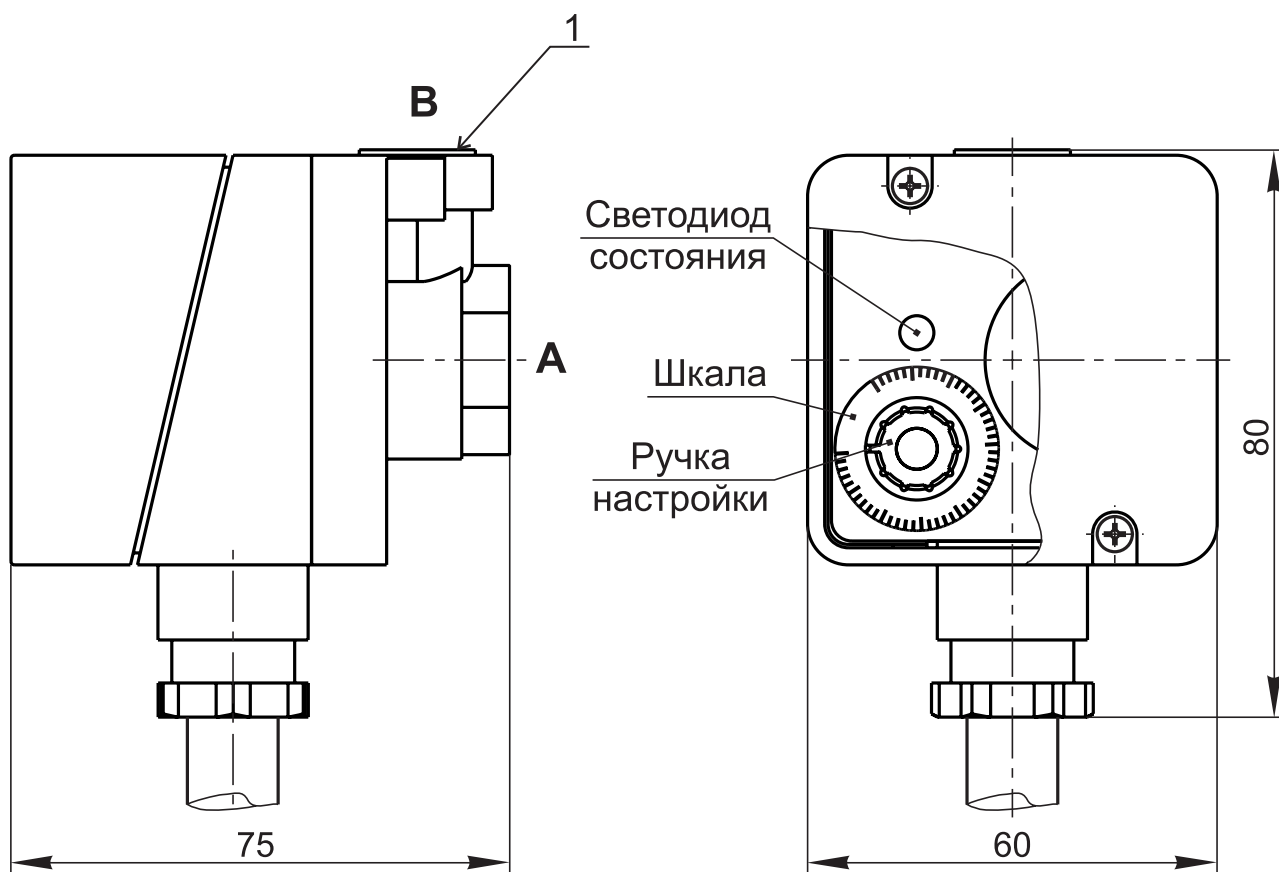
Рис. 25-5. Габаритные размеры датчиков-реле давления серии ДРД электронного типа
