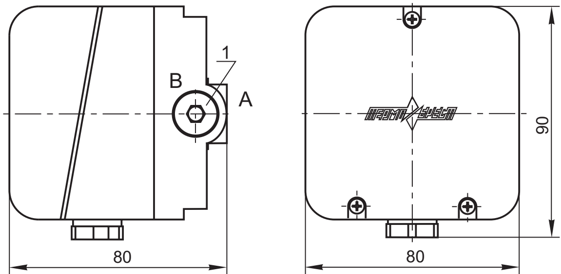
Рис. 25-2. Габаритные размеры датчиков-реле избыточного давления (напора) серии ДРД-Н
