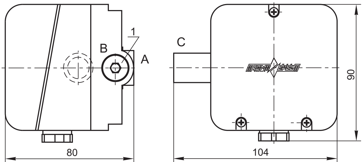
Рис. 25-3. Габаритные размеры датчиков-реле вакуумметрического давления (тяги) серии ДРД-Т
