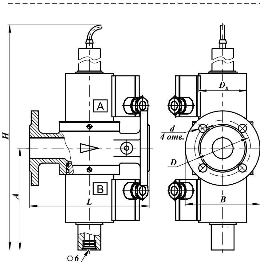
Рис. 18-5. Клапаны трехпозиционные фланцевые на DN 25 с одним регулятором расхода и датчиком положения
