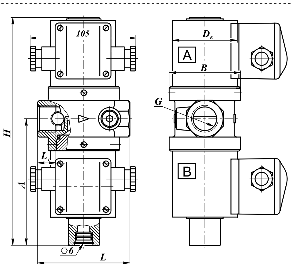
Рис. 18-1. Клапаны трехпозиционные муфтовые на DN 20, 25 с одним регулятором расхода
