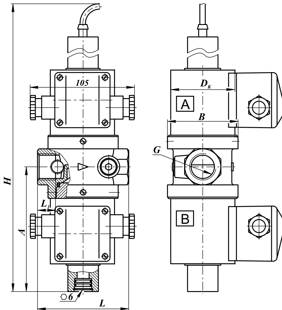
Рис. 18-2. Клапаны трехпозиционные муфтовые на DN 20, 25 с одним регулятором расхода и датчиком положения
